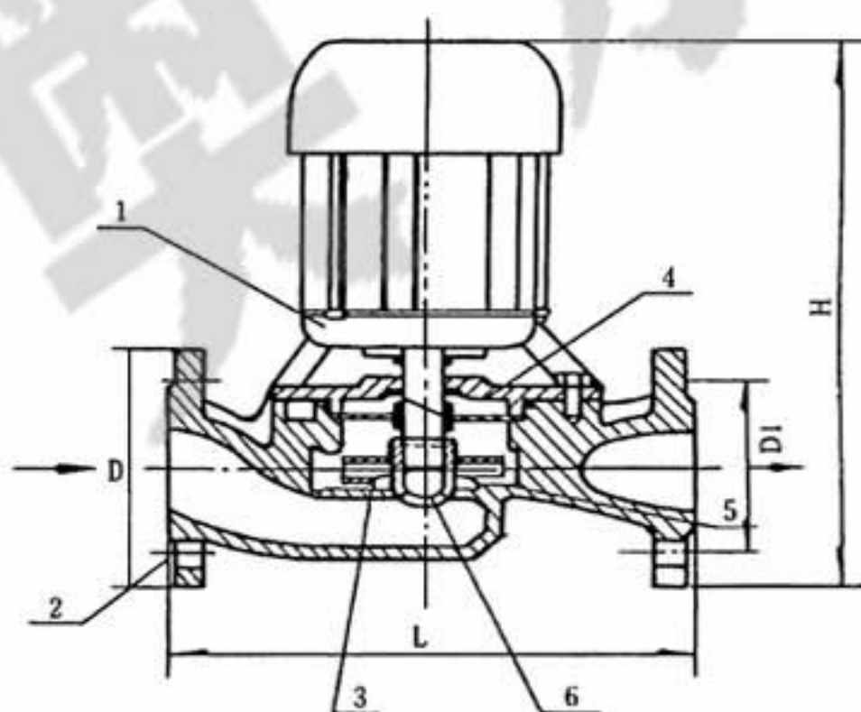
该泵法兰连接根据(JB78-59) 标准制造
